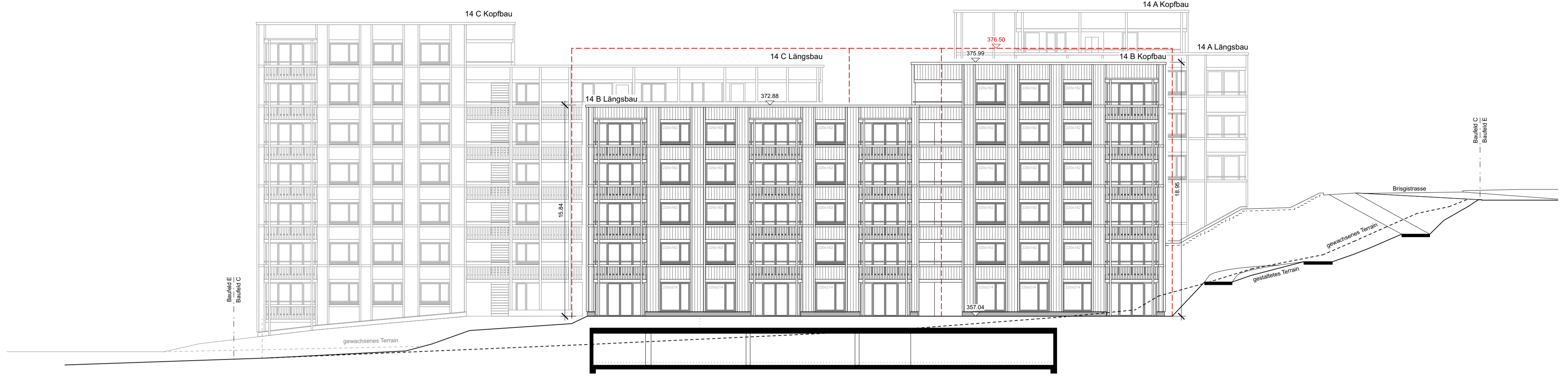
Westfassade
