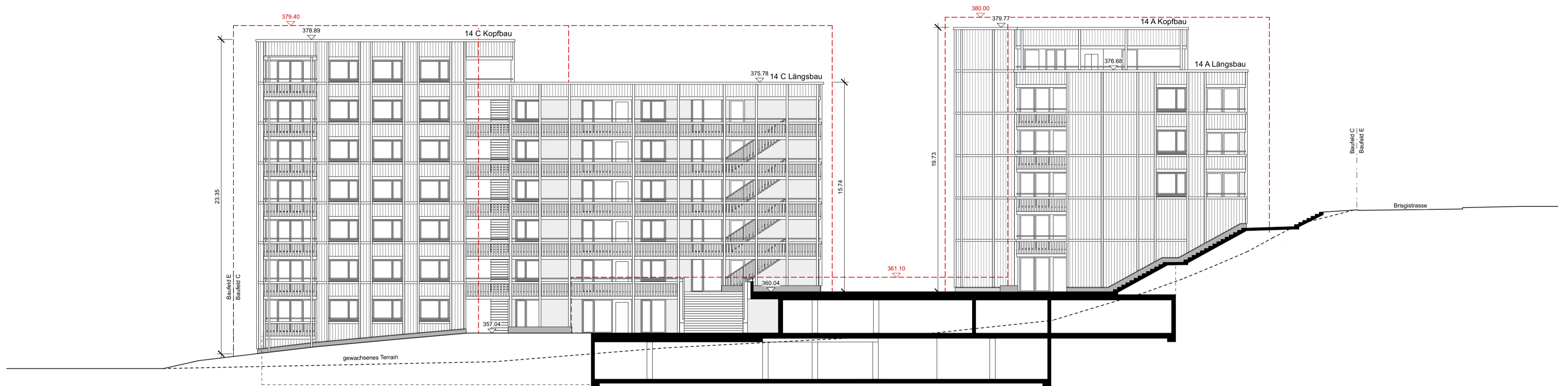
Schnitt CC
